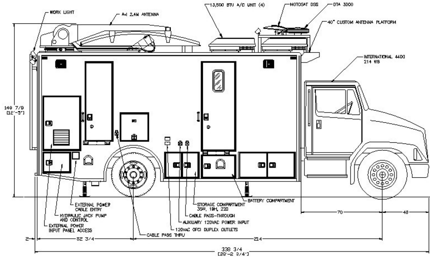
CURBSIDE ELEVATION
